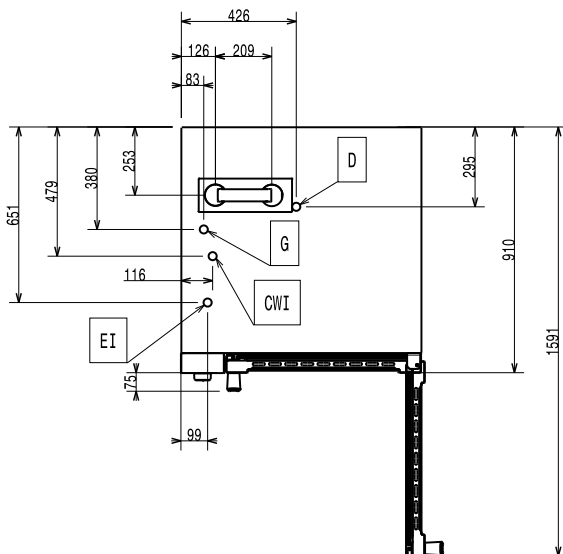
Dessus
